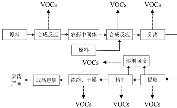
图 1-1 典型化学农药制造工艺与 VOCs 排放环节图
