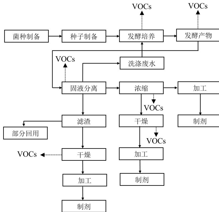
图 1-2 典型生物农药制造工艺与 VOCs 排放环节图
